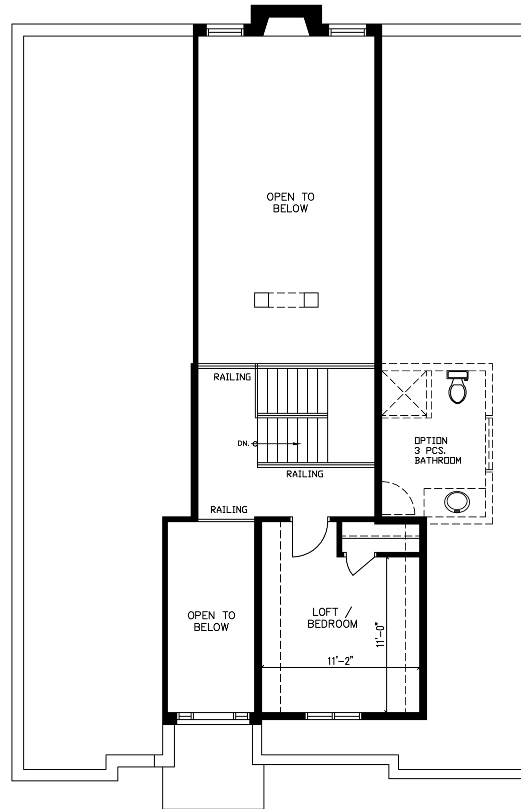
OPTIONAL LOFT FLOOR 320 sq.ft.
